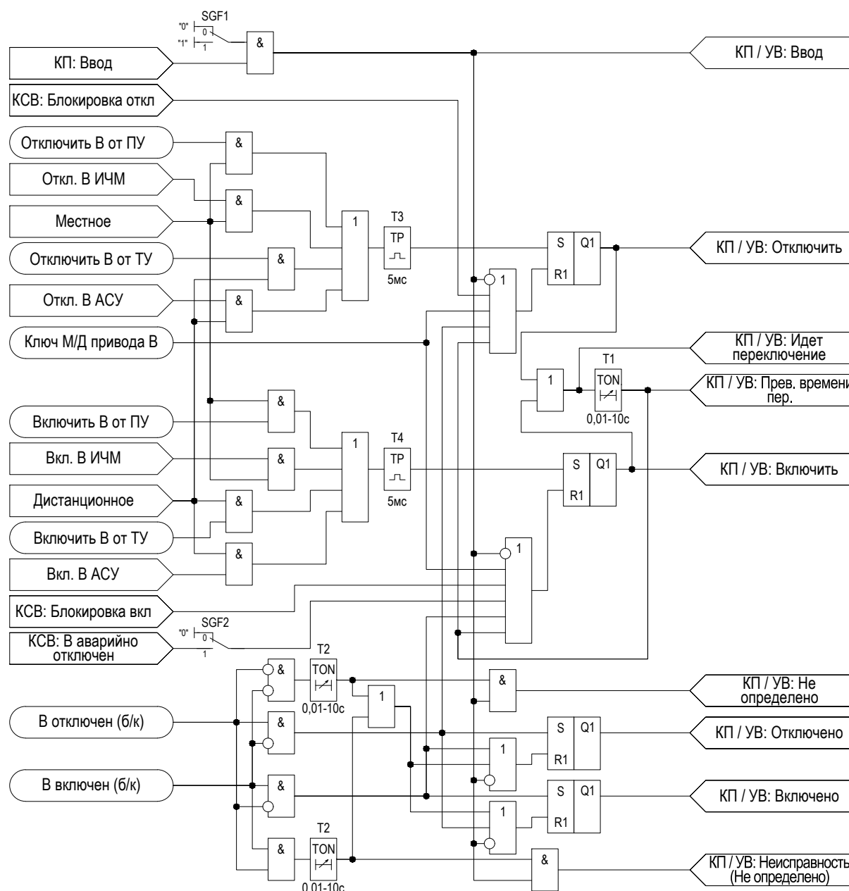
Рисунок 2.4 – Функциональная схема «УВ»
