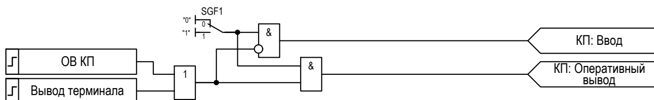
Рисунок 2.3 – Функциональная схема управления режимами работы «КП»
